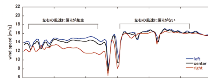
図4 シミュレーションによる風車中心高さでの風速時間変化
