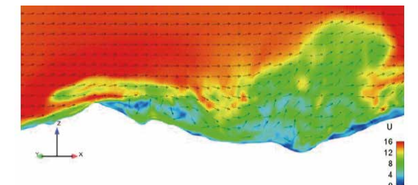
図5 風速分布 (垂直断面)
