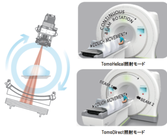
図1 トモセラピー装置
