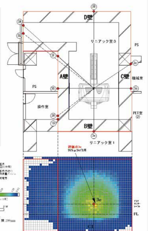
図4 B壁面での放射線量分布
