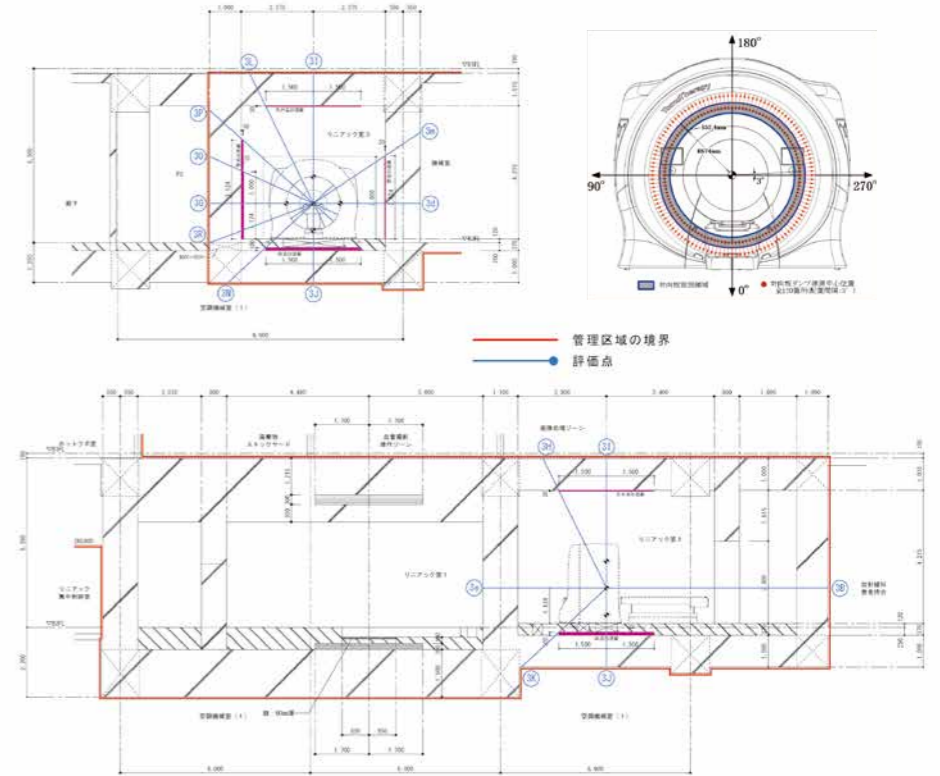
図2 トモセラピー治療施設とエックス線粒子発生装置の位置
