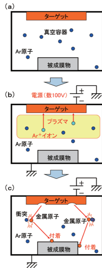
図1 スパッタ成膜のメカニズム
