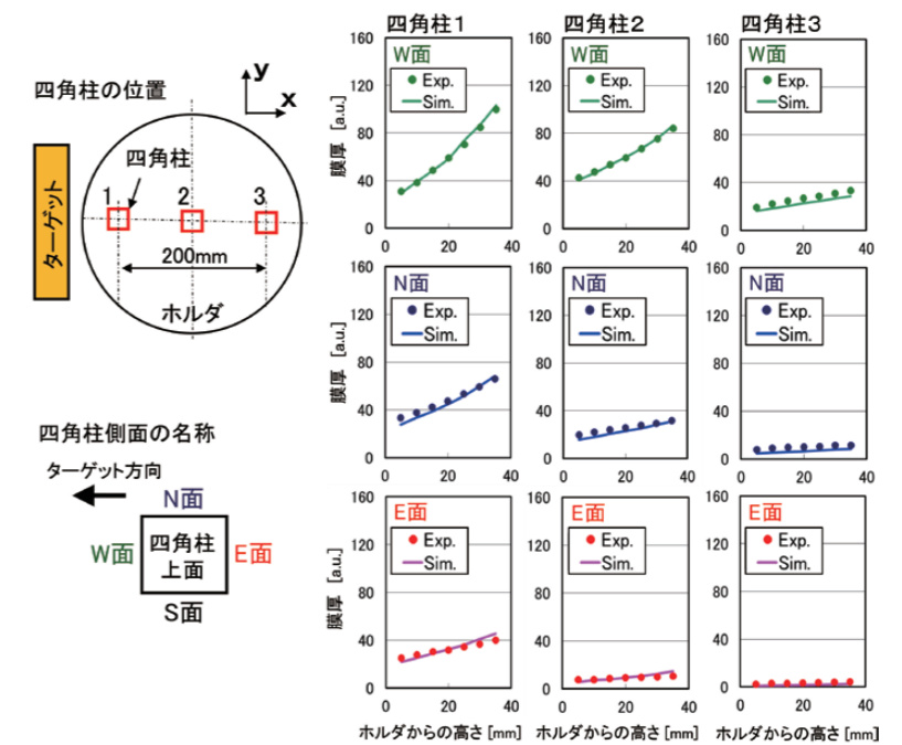
図4 実験結果と解析結果の比較
