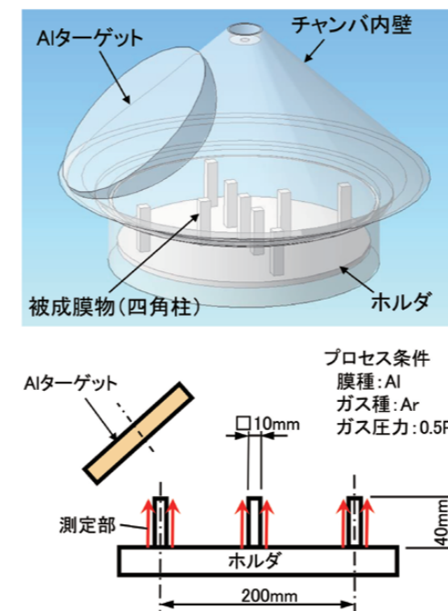
図3 装置内部と被成膜物の構造
