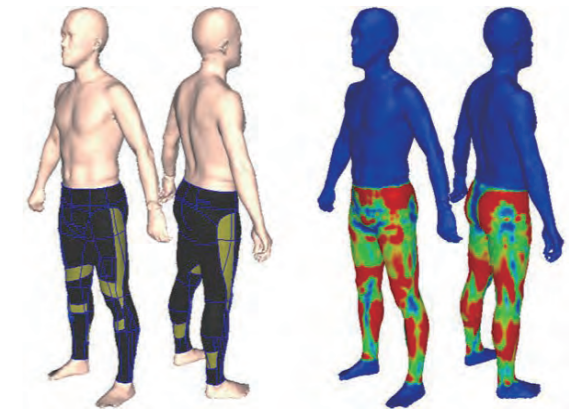
図2 シミュレーションによる装着状態の再現 (右:衣服圧の分布)
