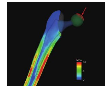
図4. 人工股関節置換の応力解析
