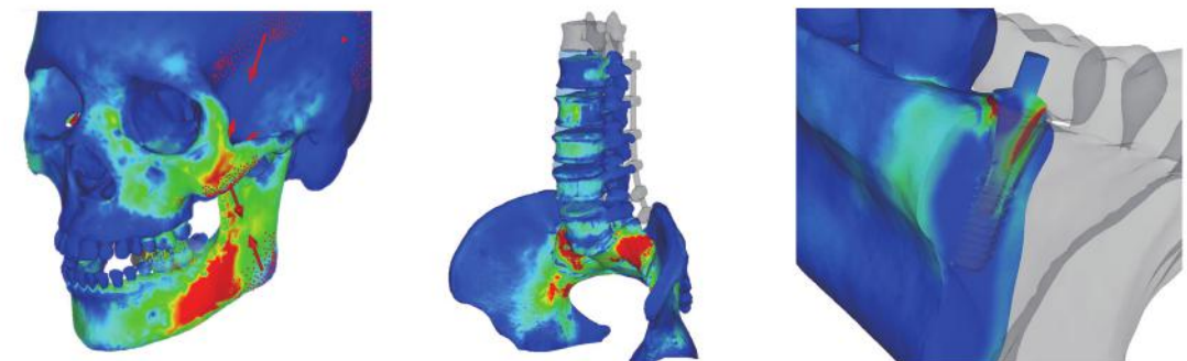
図5. 左から、咬合時の応力分布、脊椎後方固定術時の応力分布、歯科インプラント挿入時の応力分布
