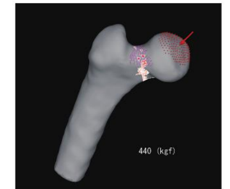
図3. 解析による頸部骨折の様子
