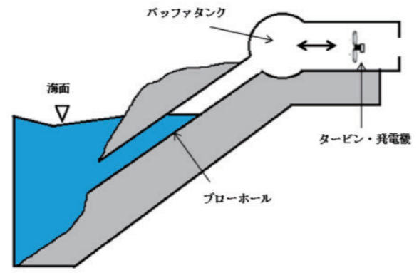
図1. 振動水柱型波力発電システム 波の上下動を振動する空気流に変換し、タービンを回して発電します。
