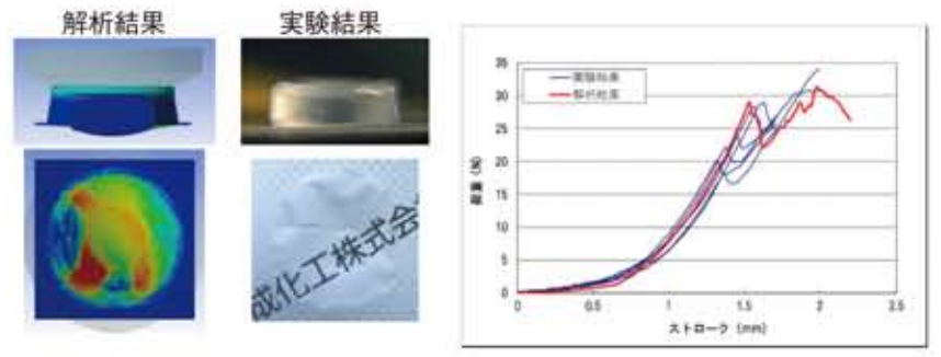
図4. 薄ポケットでの実験と解析結果の比較
