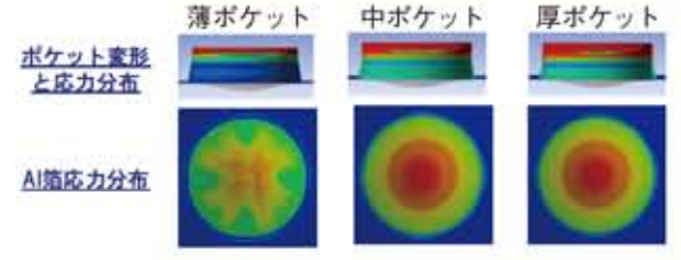
図3. ポケット厚みによる錠剤取り出しの際の応力分布
