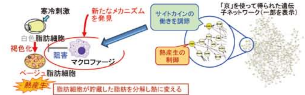
図3. 「京」を活用した大規模な遺伝子ネットワーク解析により脂肪細胞の褐色化の新たな制御メカニズムを発見
