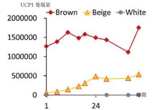
図2. uncoupling protein 1 (UCP1) の発現量の経時変化
