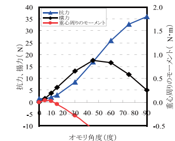
図3. 開発した鋳鉄製オモリにかかる力と重心まわりのモーメントのシミュレーション結果
