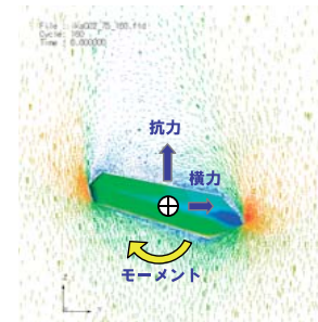
図2. 従来の鉛製オモリにかかる力と重心まわりのモーメントのシミュレーション結果
