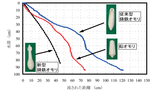
図1. 流れがある中での1/2模型の落下軌跡
