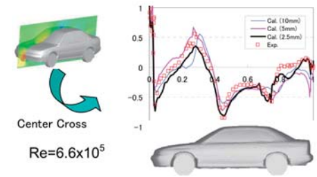
図2. 空力シミュレーションモデル
