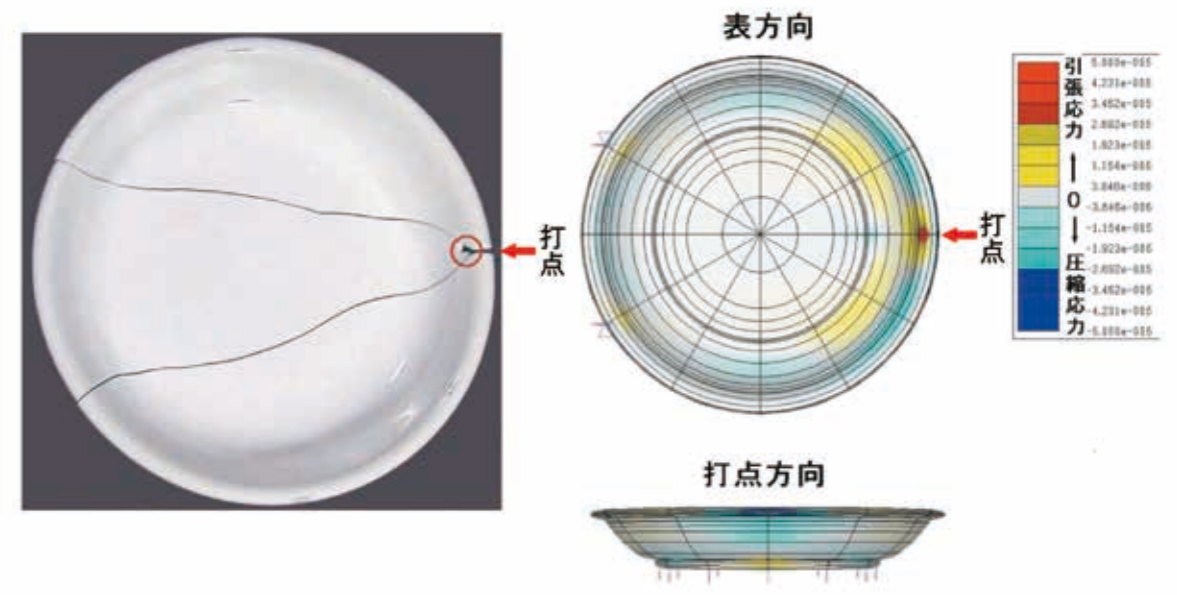
図1. 衝撃試験後の破壊状況(左)と応力シミュレーション結果(右)
